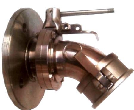
Válvula para recibir coples rápidos
